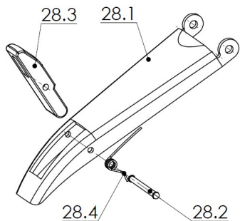
Zespół dźwigni zaworu SK125A9-60.00.0
